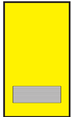
Louver 24" x 12"
